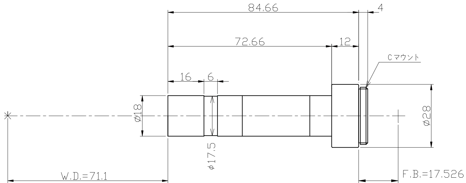
KCM-05 : 倍率=0.5倍 W.D. (作動距離)=71mm
